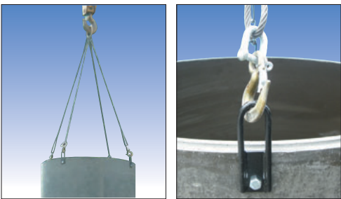
4号マンホール吊り上げ状況
