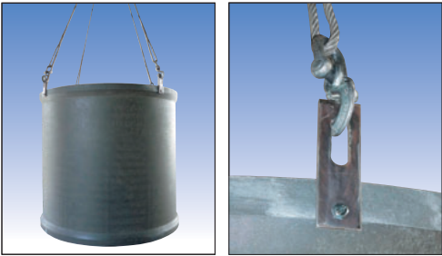
3号マンホール吊り上げ状況
